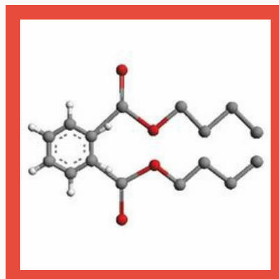
Dibutyl Phthalate
